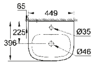
39 324 000 39 324 00H* Handrinse basin 45 cm
