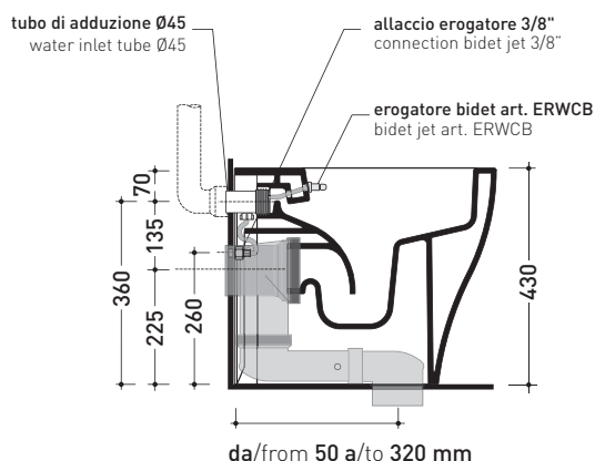
sezione longitudinale / section
